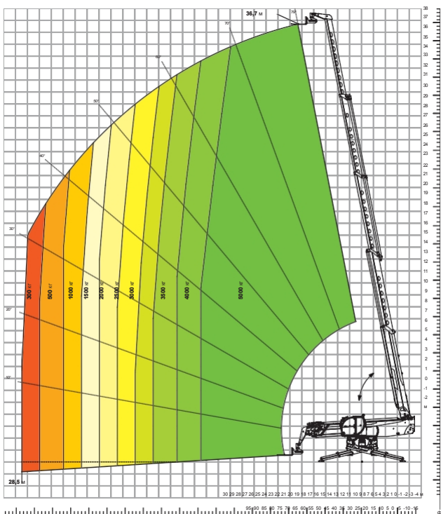
Таблиця навантажень з Обертові вила, 5000 кг ATT - 03 - 041
