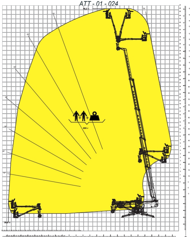
Завантажити діаграму з ПЛАТФОРМОЮ «ПОВЕРХ-ПІД» – ПОЗИТИВНОЮ ATT - 01 - 024
