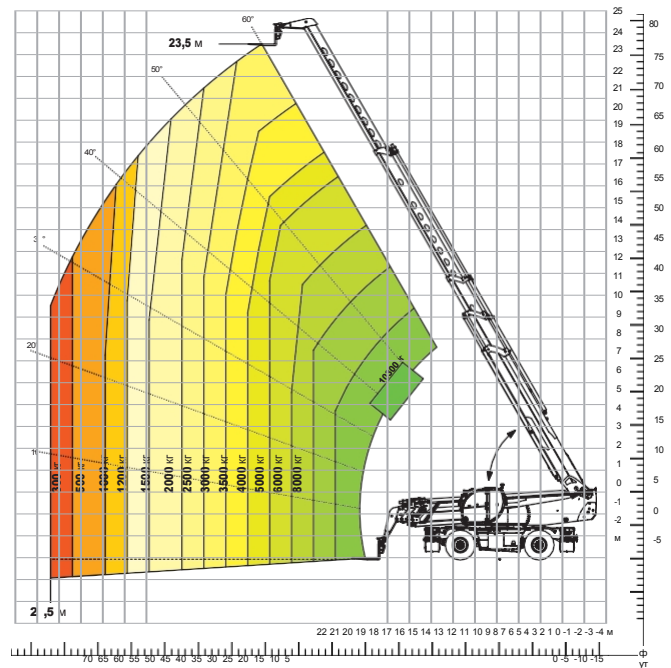
Таблиця навантажень з СТРІЛОЮ З ЛЕБЕДКОЮ, 800 кг ATT - 04 - 005
