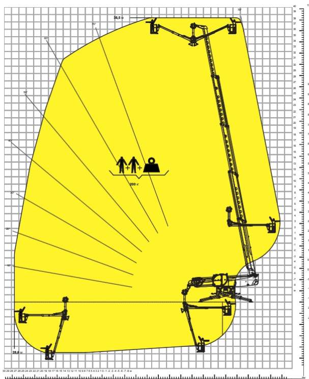
Таблиця навантажень із ПЛАТФОРМОЮ OVER-UNDER – NEGA ATT - 01 - 024
