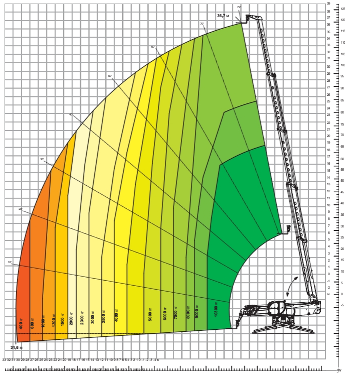
Таблиця навантажень з ПОВНІСТЮ ВИСУНЕНИМИ СТАБІЛІЗАТОРАМИ (360°) ATT - 03 - 018
