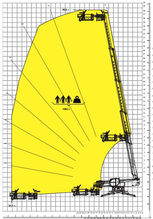
Таблиця навантажень з ВИСУВНОЮ ПЛАТФОРМОЮ ДЛЯ ДАХІВ, 1 000 кг ATT - 01 - 020
