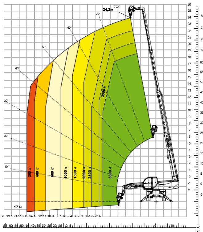
Таблиця навантажень з ЛЕБЕДКОЮ 3 500 кг АТТ - 02 - 002
