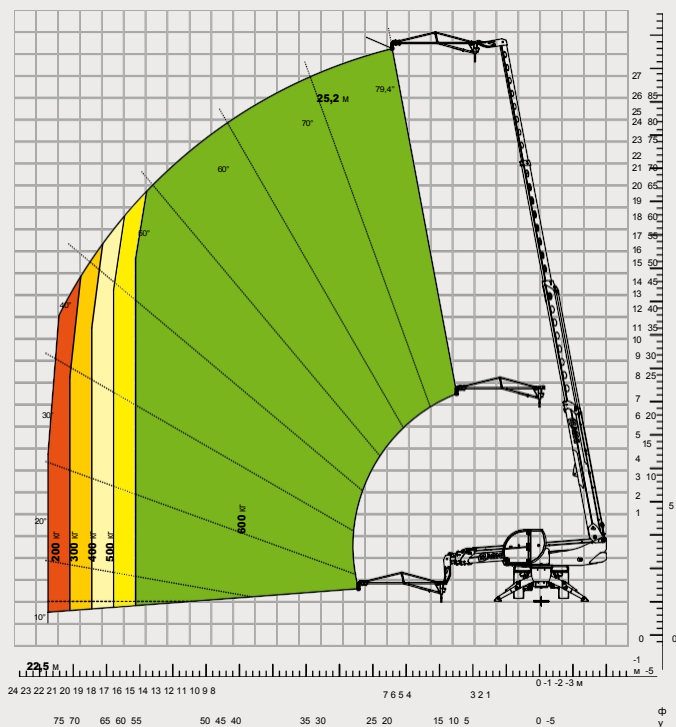
Таблиця навантажень з Поворотний кран, 600 кг АТТ - 04 - 001
