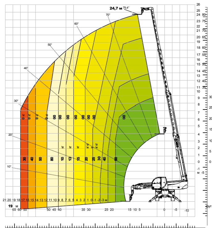
Таблиця навантажень з ЛЕБЕДКОЮ 3 500 кг АТТ - 02 - 002
