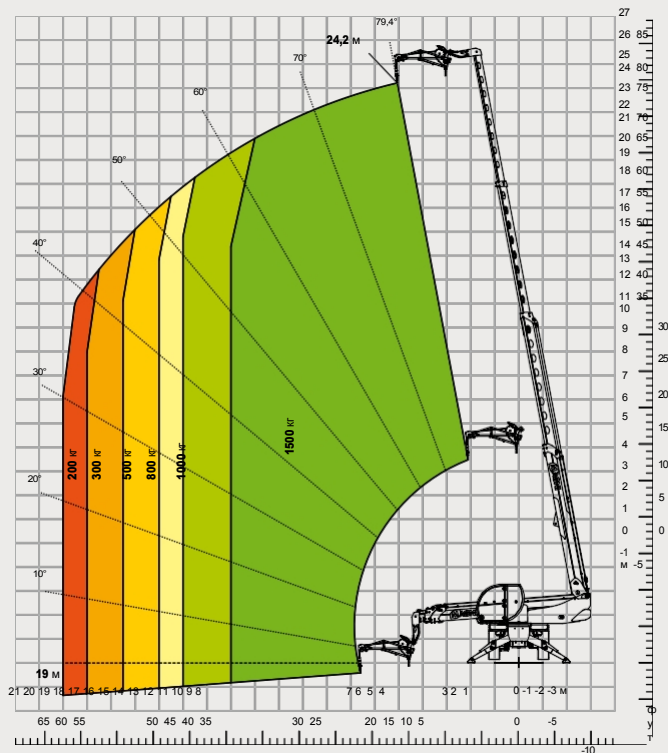
Таблиця навантажень з СТРІЛОЮ З ЛЕБЕДКОЮ, 1 500 кг АТТ - 04 - 011
