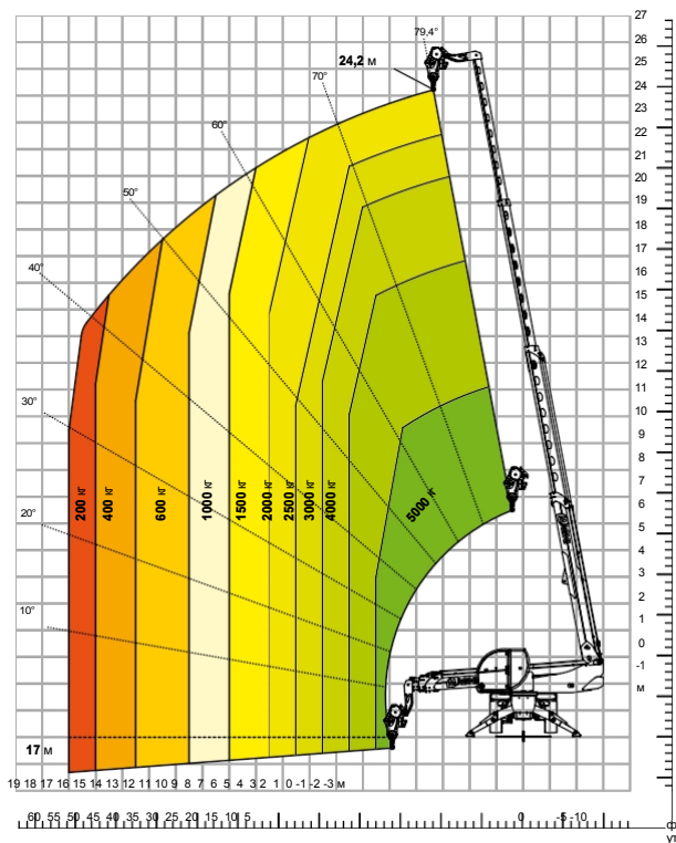
Таблиця навантажень з ЛЕБЕДКОЮ 5 000 кг АТТ - 02 - 019
