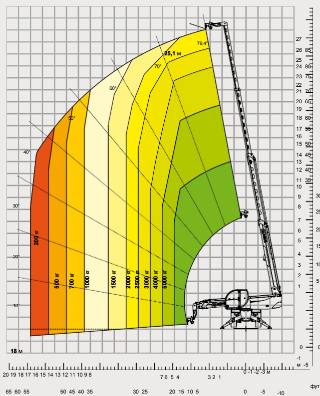
Таблиця навантажень з ГАКОМ 5 000 кг АТТ - 05 - 014
