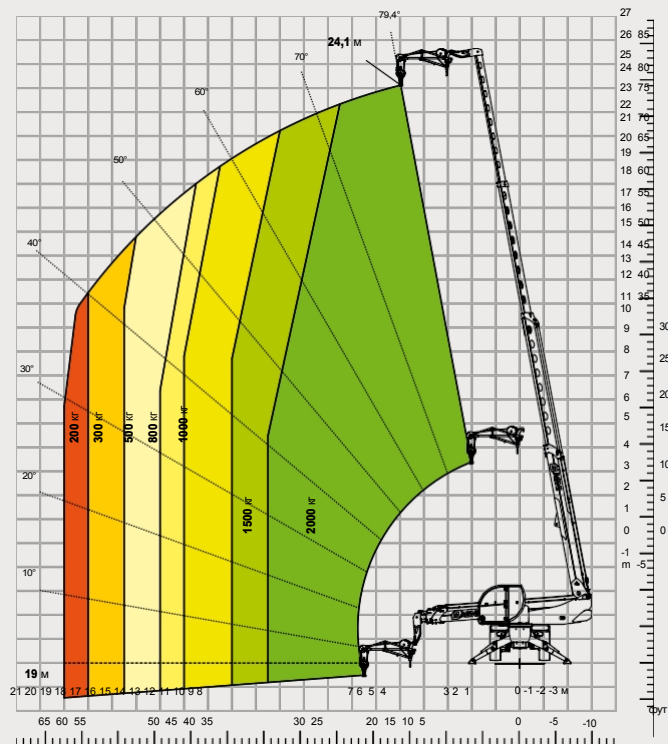
Таблиця навантажень з СТРІЛОЮ З ЛЕБЕДКОЮ, 2 000 кг АТТ - 04 - 015
