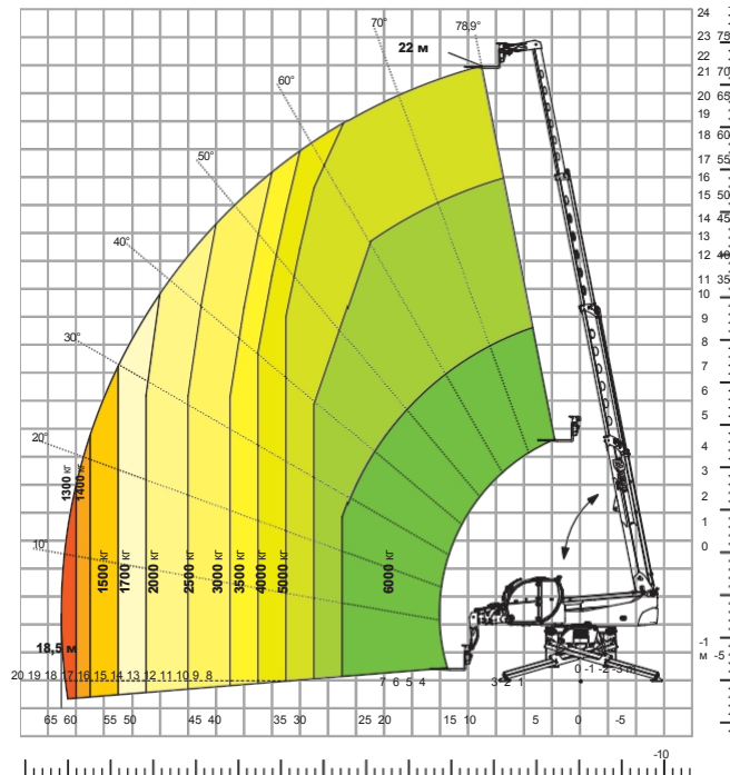
Таблиця навантажень з ЛЕБЕДКОЮ, 3 500 кг АТТ - 02 - 002
