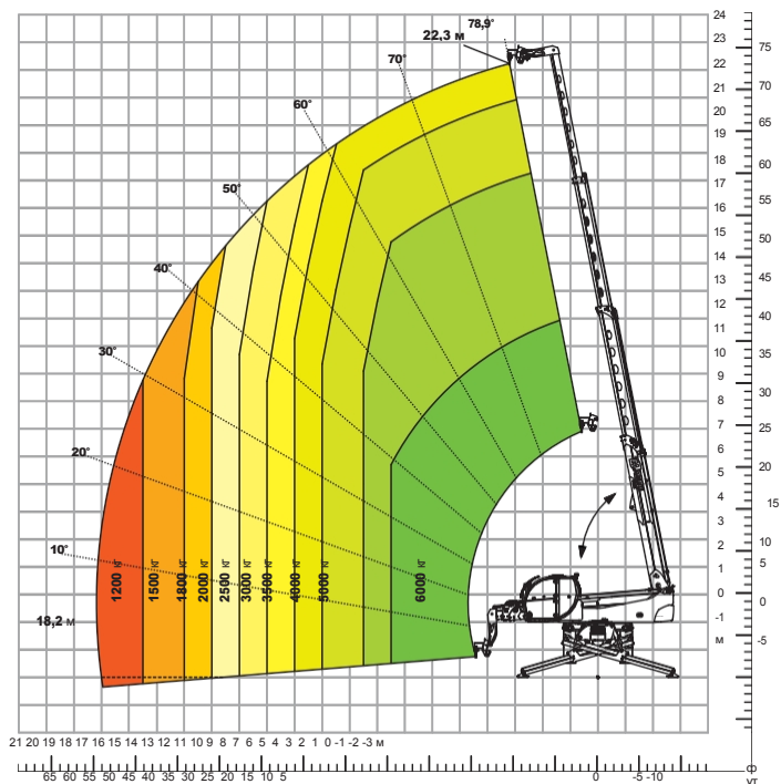
Таблиця навантажень з ОБЕРТОВОЮ ВИСУВНОЮ ПЛАТФОРМОЮ, 1 000 кг ATT - 01 - 016
