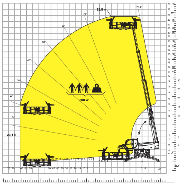
Завантажити діаграму з ПЛАТФОРМА, 500 кг, 3 ЛЕБЕДКОЮ, 600 кг ATT - 01 - 026
