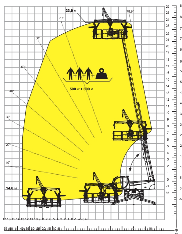
Завантажити діаграму з ПЛАТФОРМА, 500 кг, 3 ЛЕБЕДКОЮ, 600 кг ATT - 01 - 026
