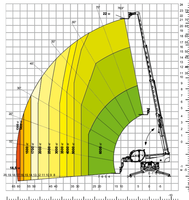
Таблиця навантажень з ЛЕБЕДКОЮ, 3 500 кг АТТ - 02 - 002
