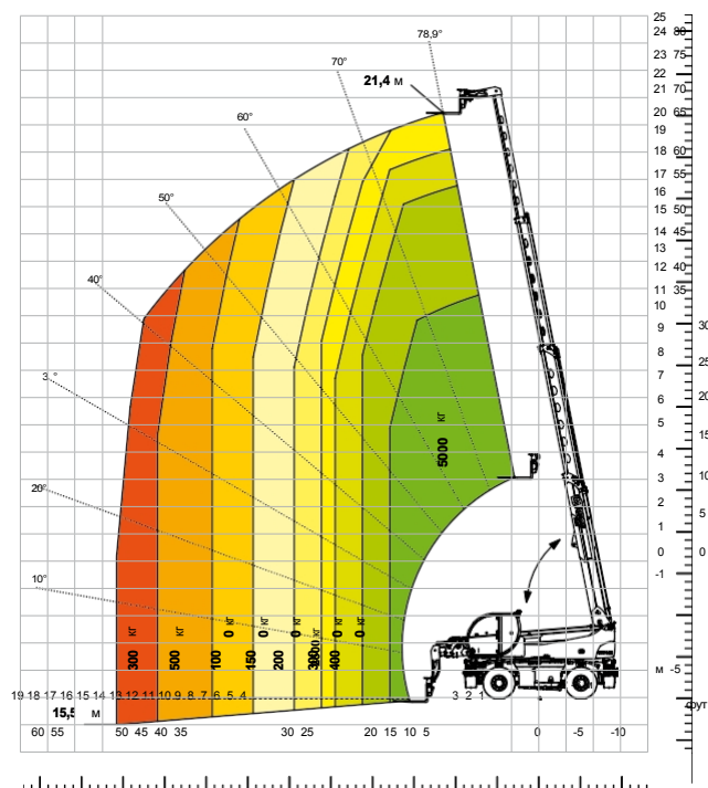
Таблиця навантажень з ЛЕБЕДКОЮ, 6 000 кг АТТ - 02 - 004
