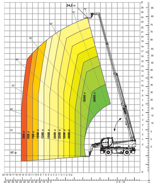
Таблиця навантажень 3 ЛЕБЕДКОЮ, 8 000 кг АТТ - 02 - 006
