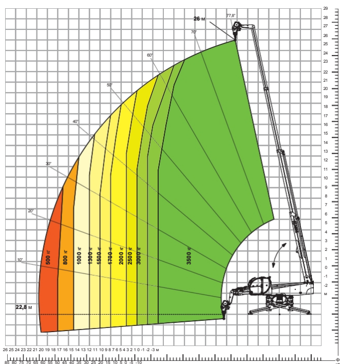
Таблиця навантажень 3 ЛЕБЕДКОЮ, 3 500 кг АТТ - 02 - 002
