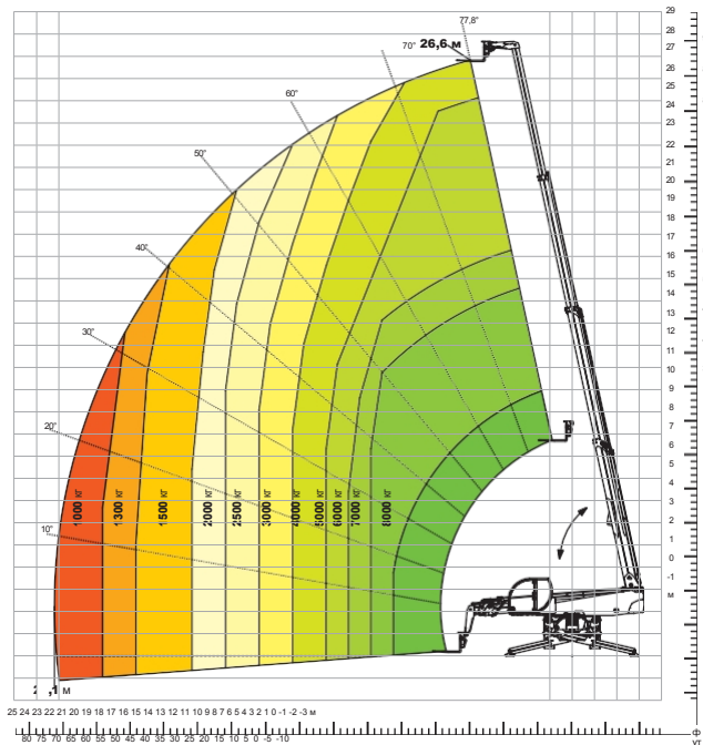
Таблиця навантажень 3 ЛЕБЕДКОЮ, 3 500 кг АТТ - 02 - 002
