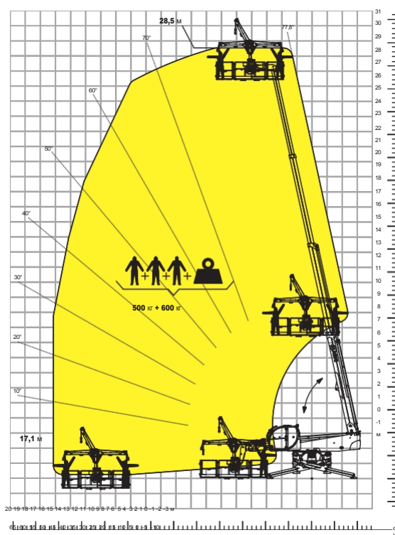
Таблиця навантажень з ПЛАТФОРМОЮ, 500 кг, з ЛЕБЕДКОЮ, 600 кг ATT - 01 - 026
