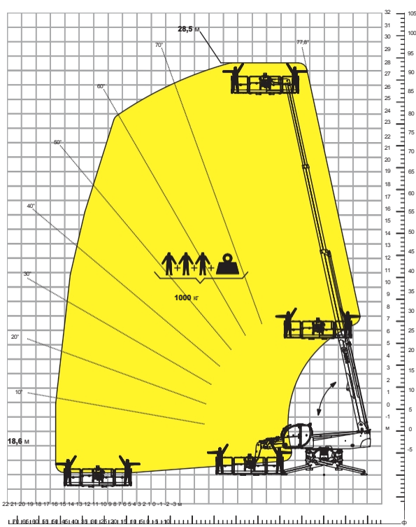
Таблиця навантажень з ОБЕРТОВОЮ ВИСУВНОЮ ПЛАТФОРМОЮ, 1 000 кг ATT - 01 - 016
