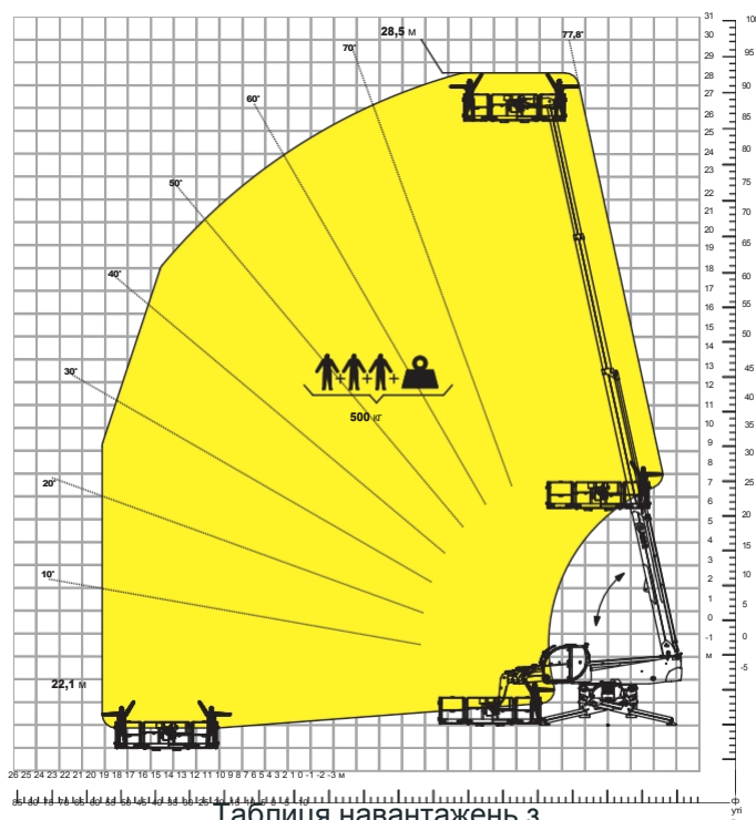
Таблиця навантажень з ПЛАТФОРМОЮ, 500 кг, з ЛЕБЕДКОЮ, 600 кг ATT - 01 - 026
