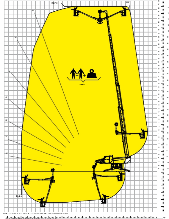
Таблиця навантажень з ПЛАТФОРМОЮ «ПОВЕРХ-ПІД» – НЕГАТИВНОЮ ATT - 01 - 024
