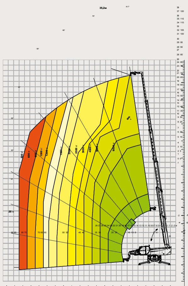
Таблиця навантажень з ГАКОМ, 8 000 кг – М1 АТТ 05 - 003
