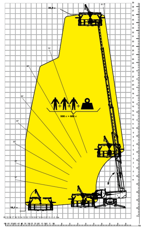
Таблиця навантажень з ПЛАТФОРМОЮ «ПОВЕРХ-ПІД» – НЕГАТИВНОЮ ATT - 01 - 024
